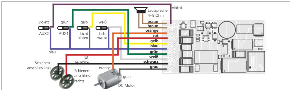
Abbildung 4: Allgemeines Anschlussschema LokSound V4.0 (Beispielverdrahtung)
