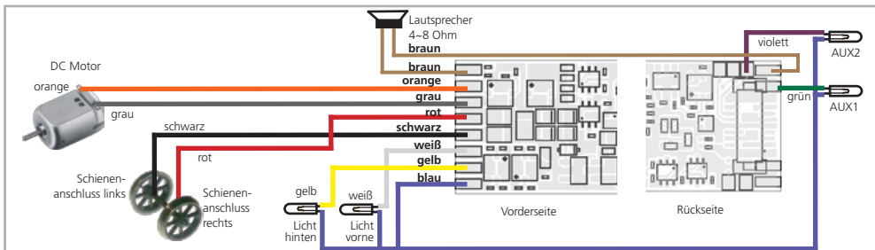
Abbildung 5: Allgemeines Anschlussschema LokSound micro V4.0 (Beispielverdrahtung)
